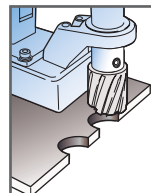
Edge hole cutting
